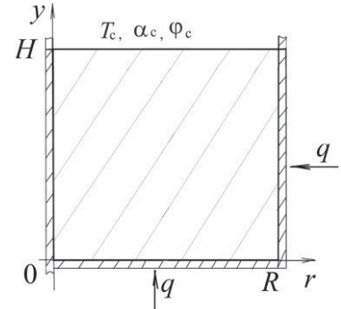
Рисунок.2 Розрахункова область
