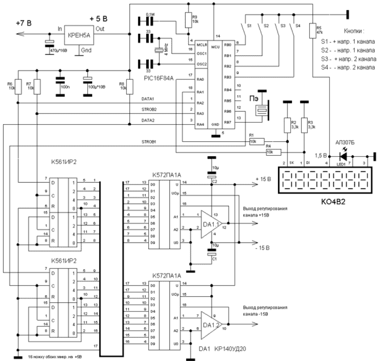
Рис. 1.14 - Контроллер регулируемого блока живлення
