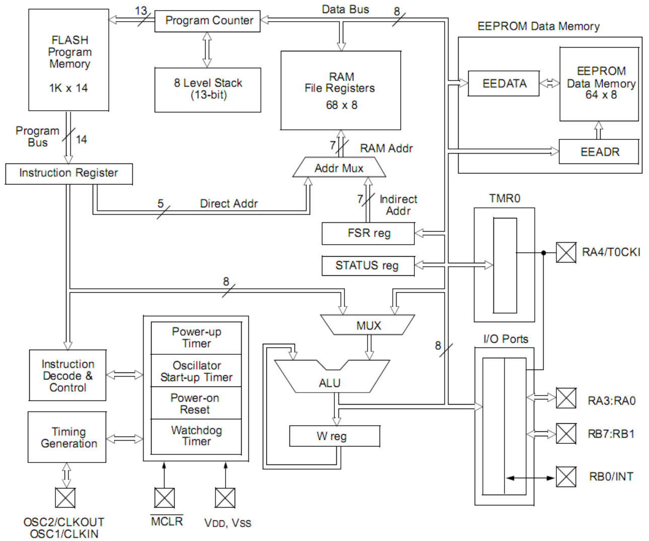
Рис. 1.7 – Архітектура мікроконтролера PIC16 F84A
