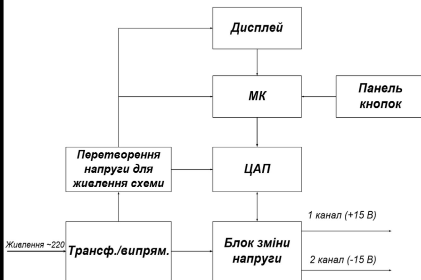
Блок- схема ІБЖ
