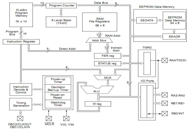
Архітектура MKC PIC16 F84A
