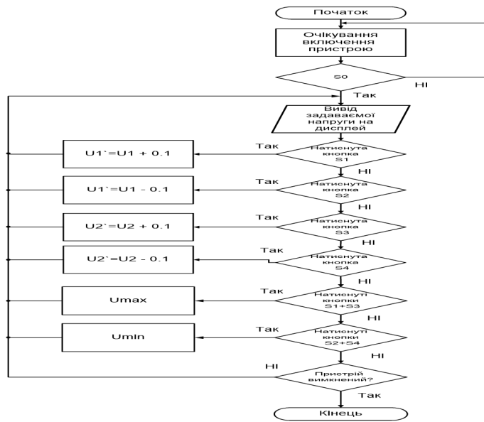
Схема алгоритму роботи ІБЖ
