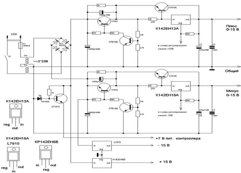
Стабилизатор блока живления + - 15В
