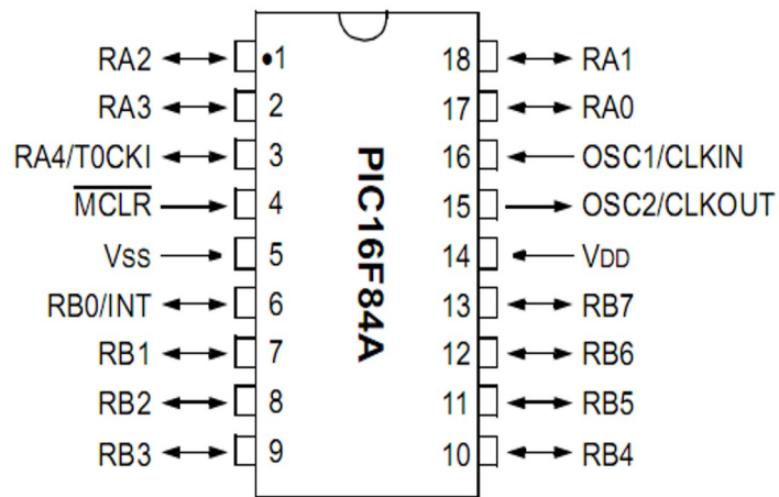
УГО MKC PIC16 F84A
