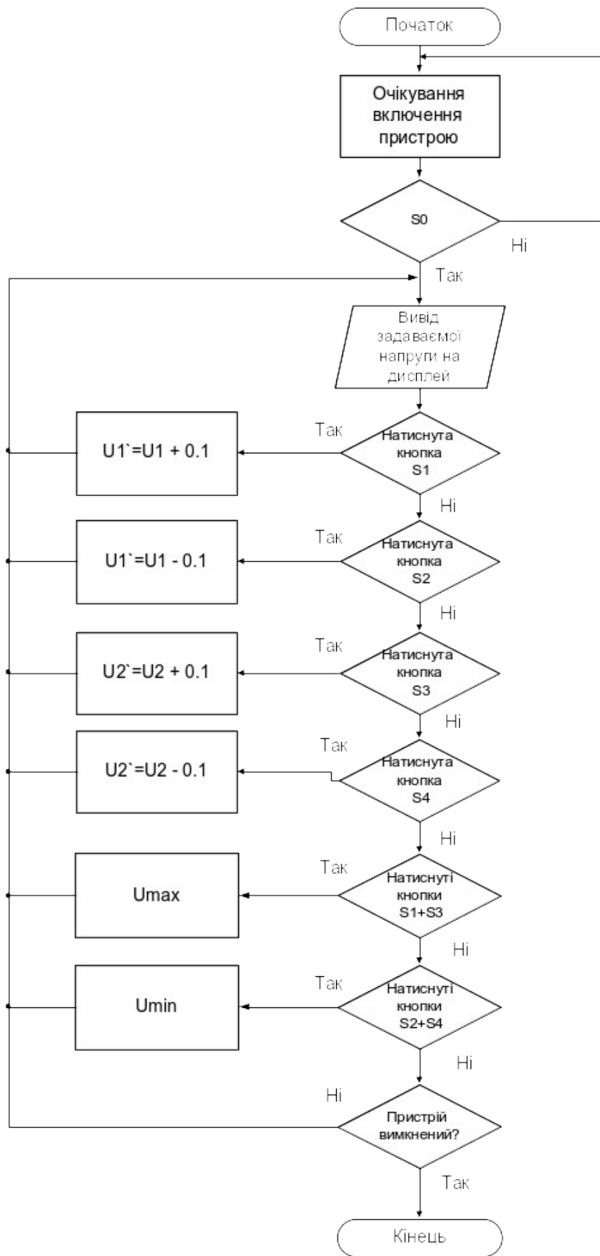
Рис. 1.17 - Схема алгоритму
