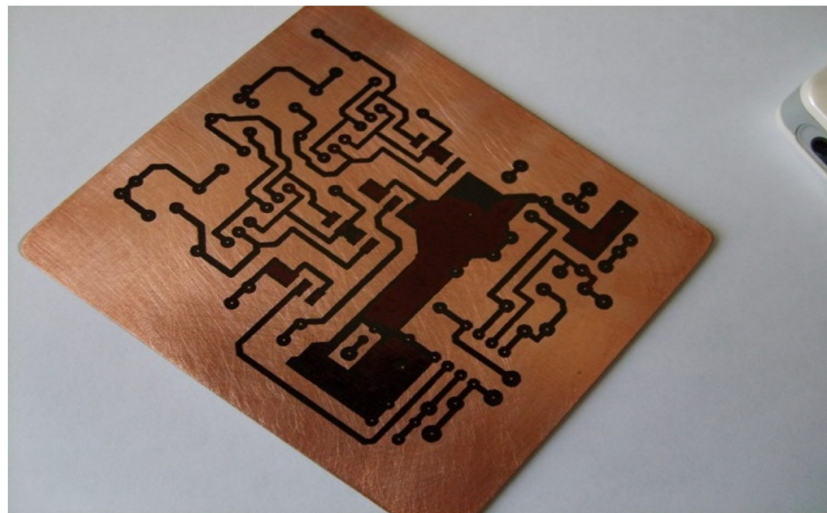
Друкована плата
