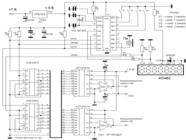
Контроллер регулируемого блока живления
