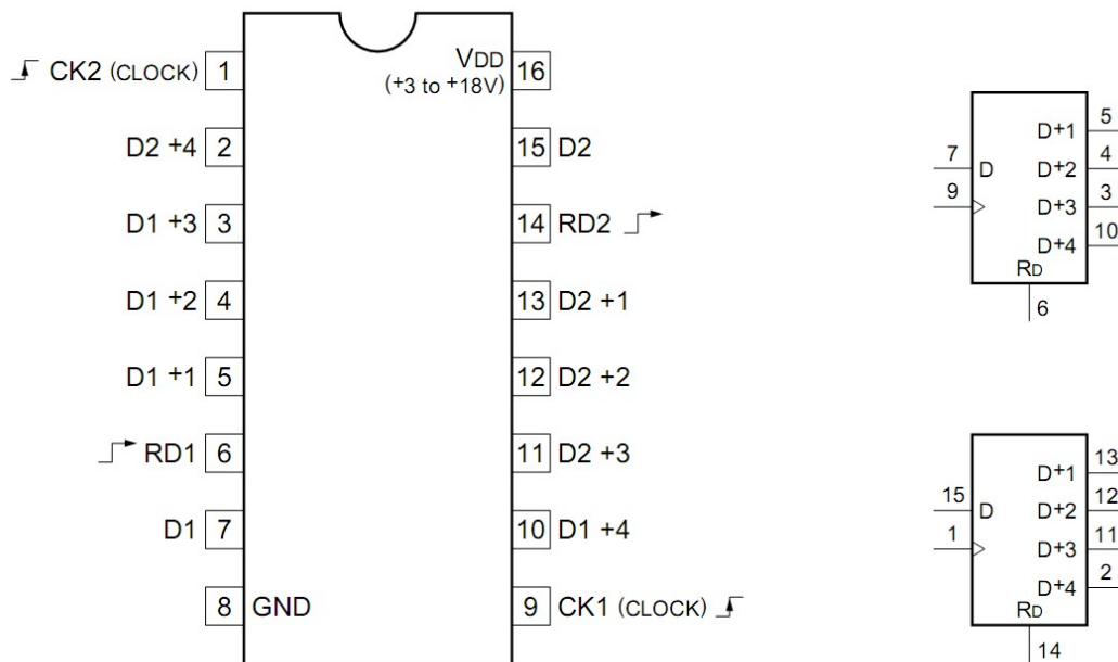
Рис. 1.12 - Мікросхема К561ІР2
