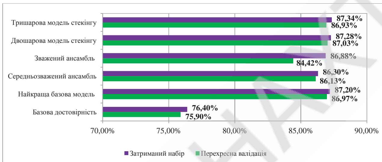
Рисунок 1 – Порівняльна характеристика розроблених моделей прогнозування
