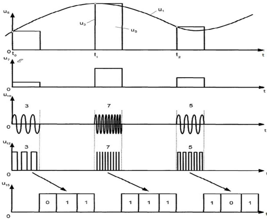
Часова діаграма перетворення аналогових сигналів на базі АДІКМ
