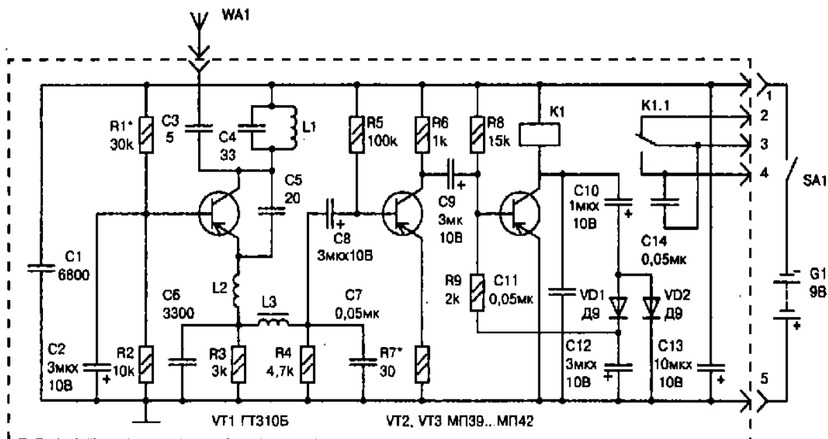
Рисунок 1.16 Схема височастотного передавача
