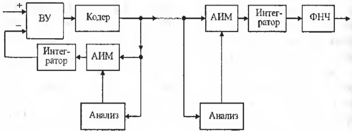
Рисунок 1.10 – Структурна схема адаптивної дельта-модуляції
