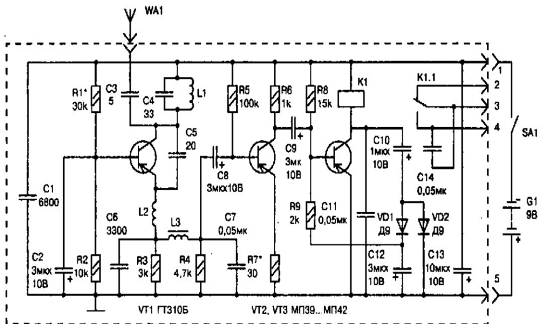
Схема высокочастотного передатчика
