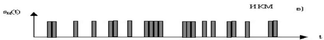
Процес дискретизації, квантування та кодування аналогового сигналу методом ІКМ
