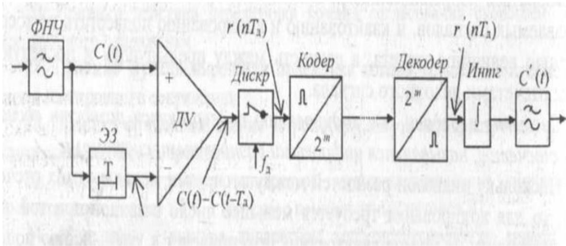
Структурна схема кодера ДІКМ: а) – кодер, б) – декодер
