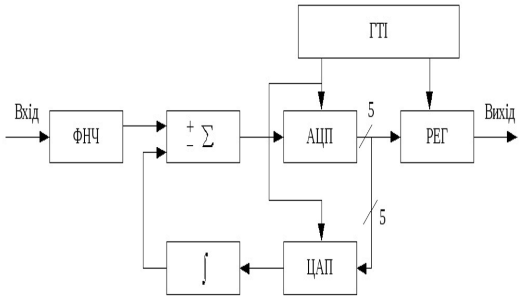
Структурна схема АДІКМ
