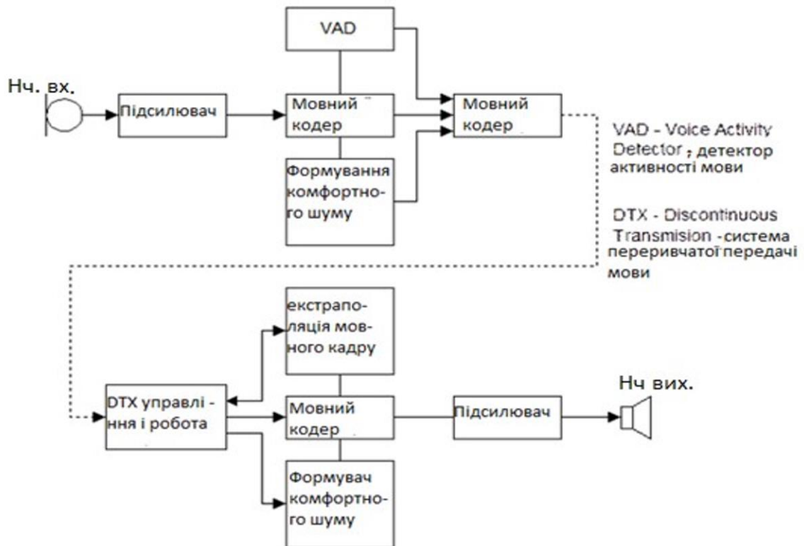
Структурна схема процесів обробки мови в стандарті GSM
