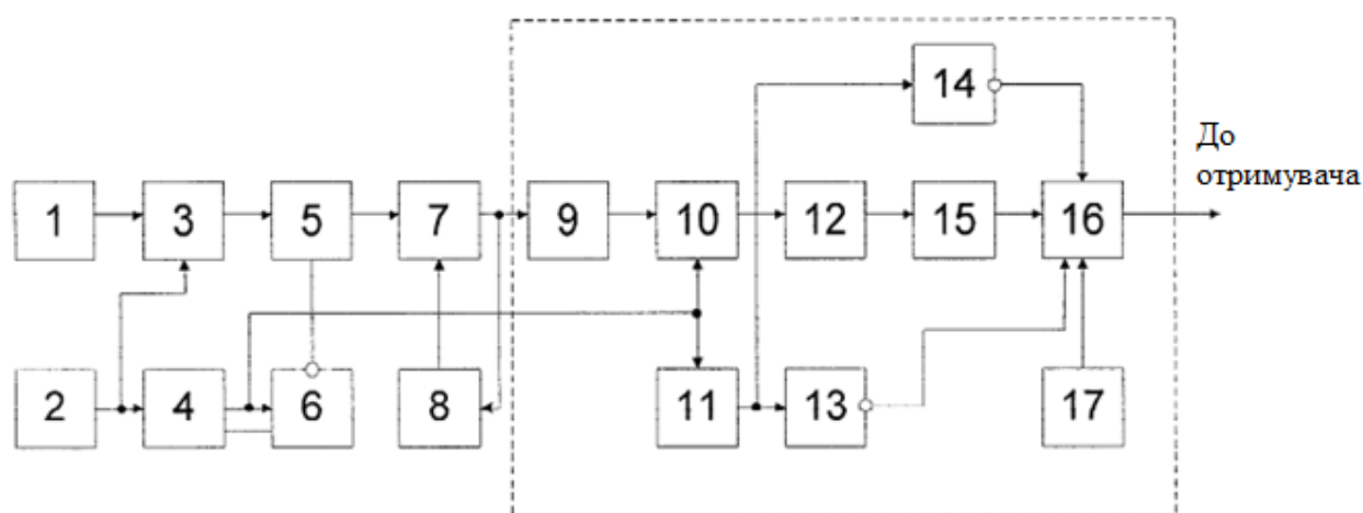
Рисунок 1.12. Структурна схема перетворювача сигналів мовлення на базі АДІКМ
