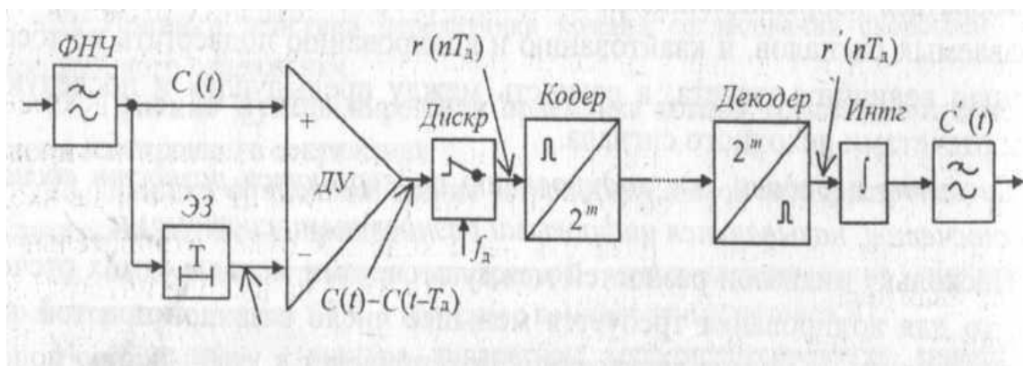
Рисунок 1.5 - Структурна схема кодера ДІКМ:
