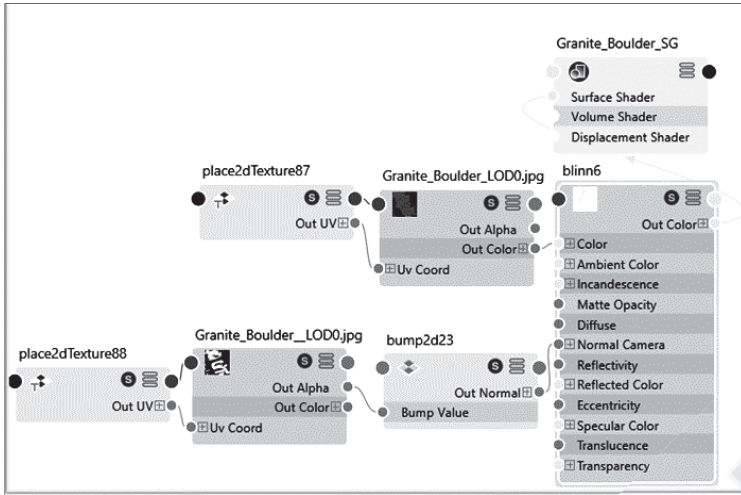
Рис. 1 – Відображення зв'язків вузлів матеріалу місячного ґрунту у Гіпершейдері
