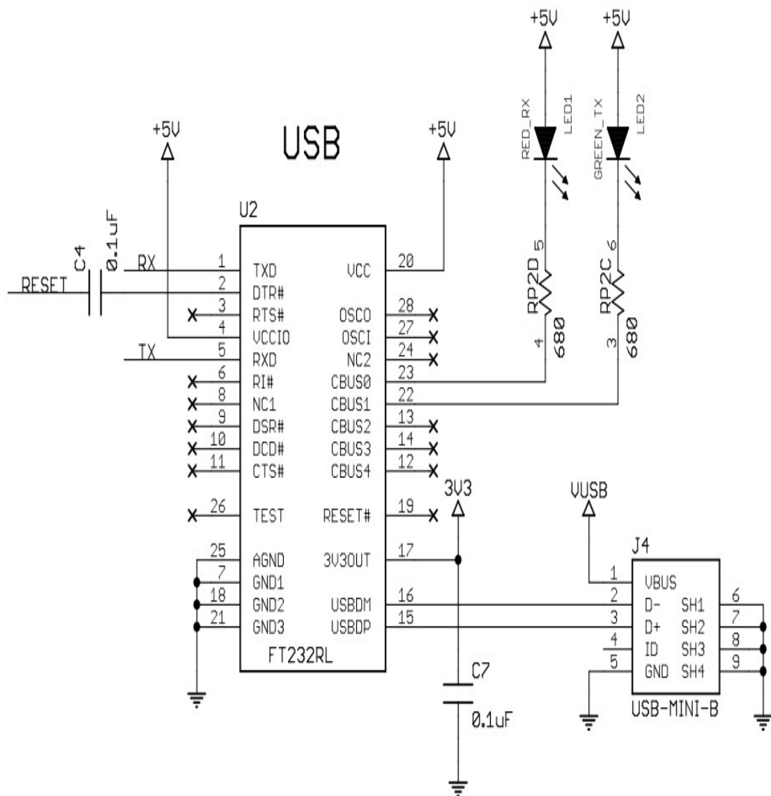
Рис. 1.10 – Принципова схема конвертора USB FT232RL
