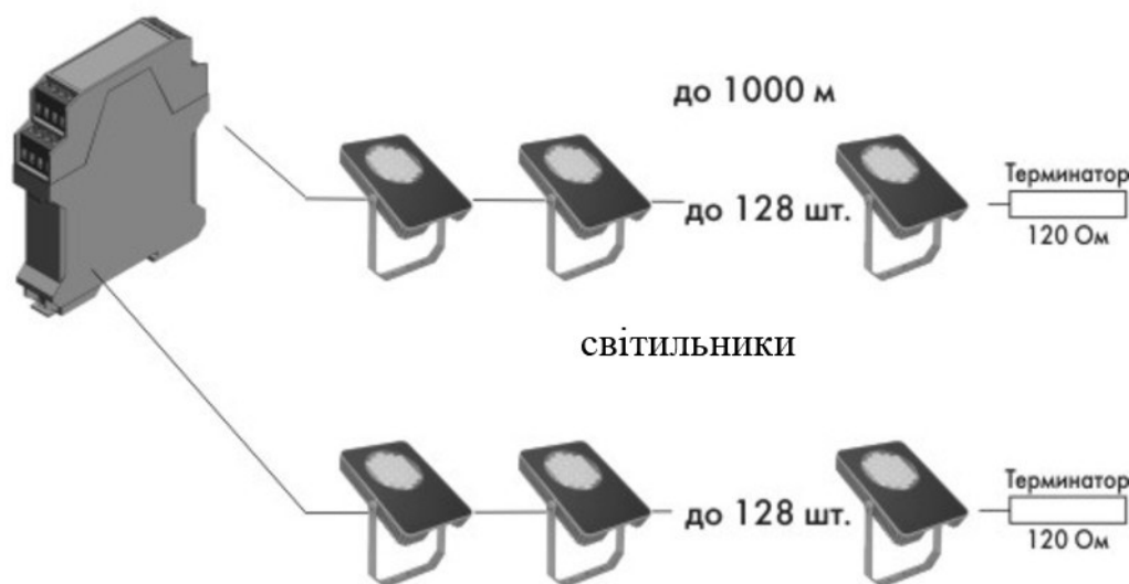
Рис. 1.6 – Система управління на базі контролера "РОНДО".
