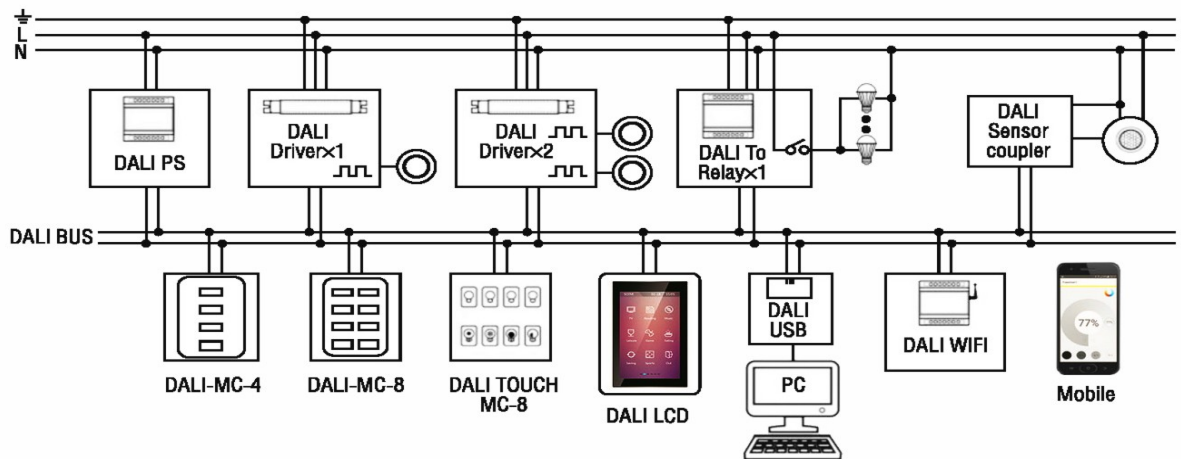
Рис. 1.2 – Управління освітленням по цифровій схемі
