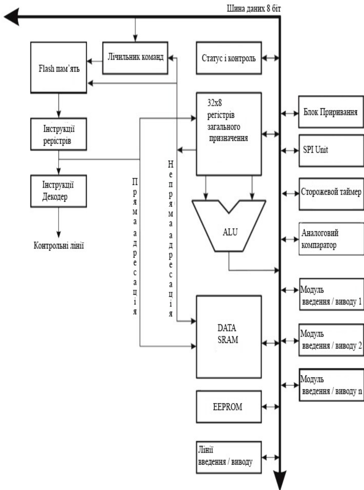
Рис. 1.7 – Блок-схема мікроконтролера ATMEGA328P
