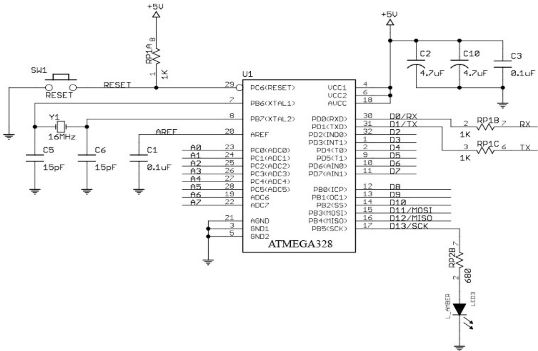
Принципова схема мікроконтролера ATMEGA 328
