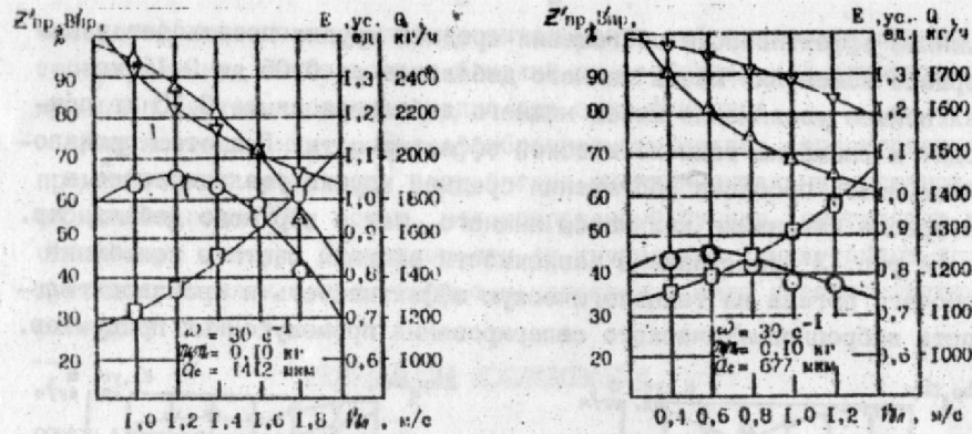
Фиг. 4. Влияние скорости восходящего воздушного потока на технологическую эффективность и производительность, а - крупная крупка; б - мелкая крупка; □ - производительность (Q); ○ - технологическая эффективность (E); Δ - относительный выход проходowego продукта (Bпр); ▽ - относительная зольность проходowego продукта (Zпр).
