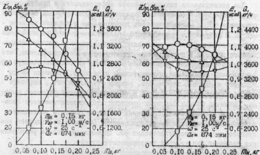
Рис. 2. Влияние массы верхнего и нижнего дебалансов на технологическую эффективность и производительность обогащения средней крупки: □ - производительность (Q); ○ - технологическая эффективность (E); Δ - относительный выход проходowego продукта (Bпр); ▽ - относительная зольность проходowego продукта (Zпр).
