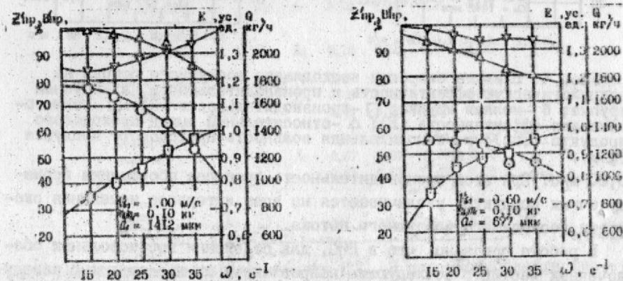
Рис. 3. Влияние частоты колебаний рабочего органа на технологическую эффективность и производительность, а - крупная крупка; б - мелкая крупка; □ - производительность (Q); ○ - технологическая эффективность (E); Δ - относительный выход проходowego продукта (Bпр); ▽ - относительная зольность проходowego продукта (Zпр).
