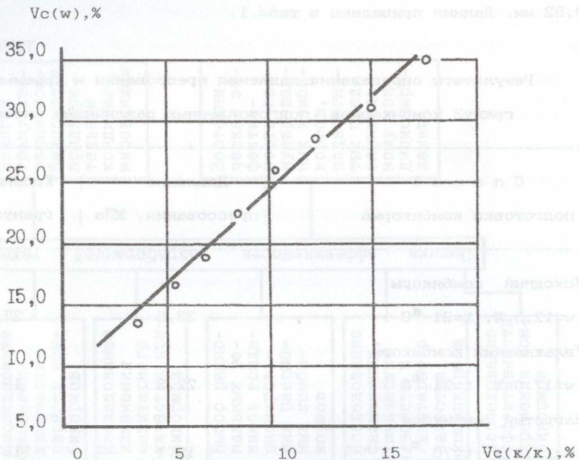
Рис.2. Зависимость коэффициента неоднородности распределения влаги в пропаренном комбикорме ( V_{cw} ) от его неоднородности по составу ( V_c к/к).
