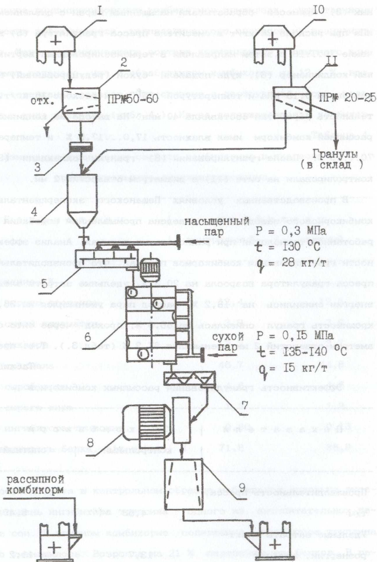
Рис.5. Схема технологического процесса гранулирования комбикормов с предварительным кондиционированием: I, IO- нория; 2- скальператор; 3- магнитный сепаратор; 4- бункер; 5- смеситель; 6- кондиционер; 7- питатель; 8- пресс-гранулятор; 9- охладитель; II- просеиватель
