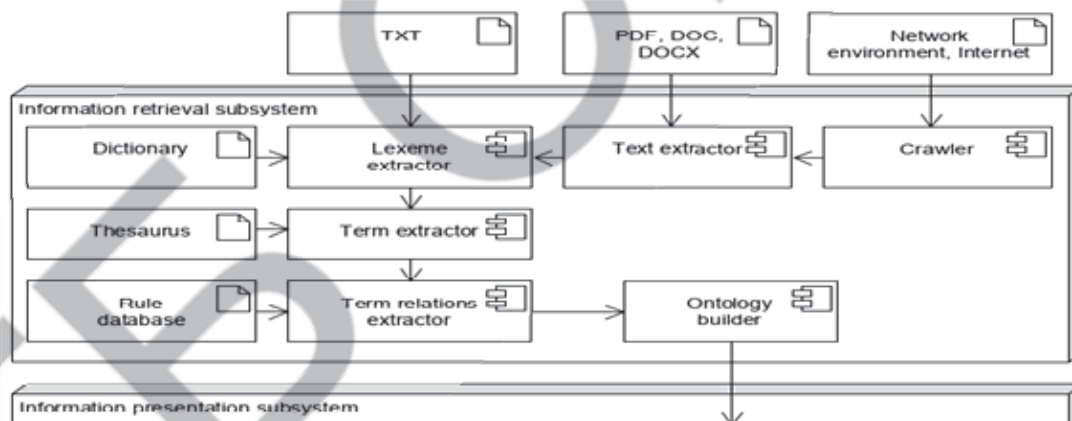
Рис. 1. Архітектура онтологокерованої Л-системи
