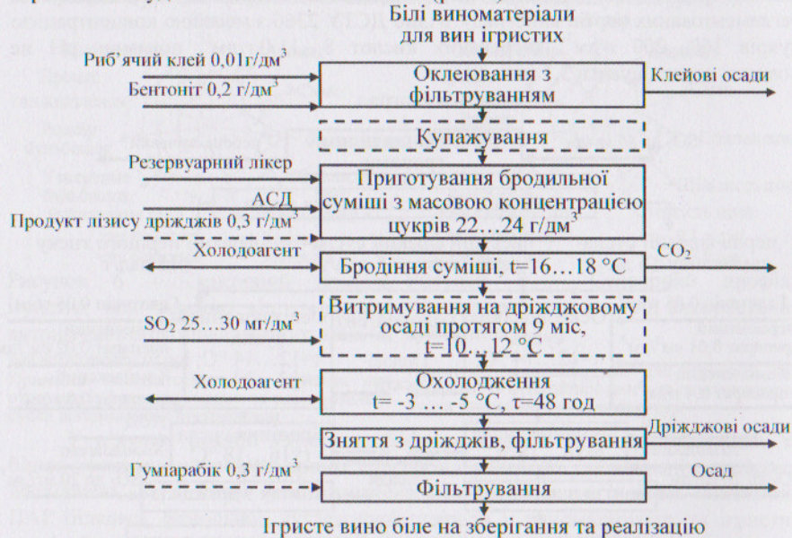
Рисунок 9 – Удосконалена принципова технологїчна схема виробництва їгристого вина бїлого резервуарним способом з підвищеними їгристими властивостями
