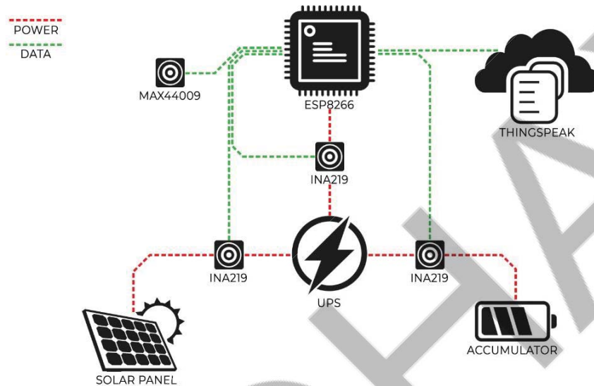
Рисунок 1 – Структурно-функціональна схема блоку автономного живлення комп'ютеризованої інформаційно-вимірювальної системи моніторингу ґрунто-кліматичних параметрів
