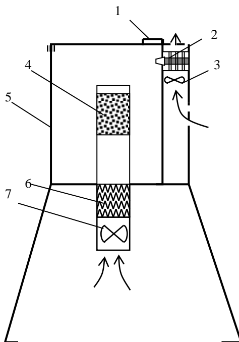
Рис. 3.1. Схема установки для исследования кинетики сушки зерновых материалов при микроволновом и конвективном нагреве.
