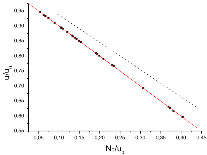
Рис. 2. Обобщающая зависимость безразмерного влагосодержания от комплекса \frac{N\tau}{u_0} для различных способах подвода теплоты.
