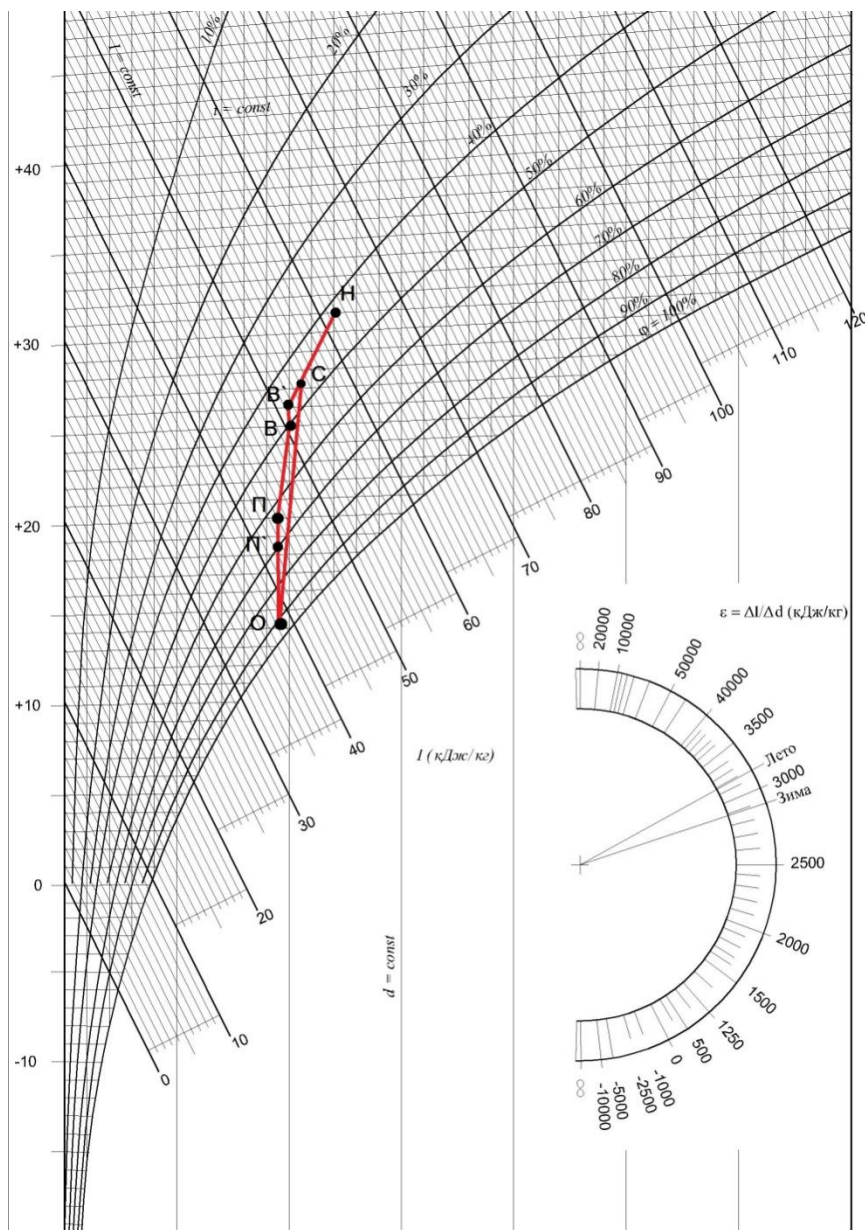
Рис.2 Процеси в ТПР
