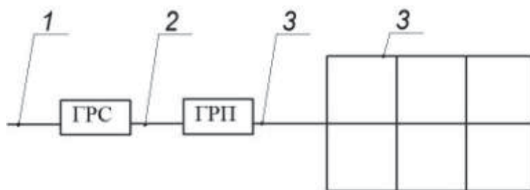
Рис. 1. Принципова схема системи газопостачання низького тиску з ГРП: 1 – газопровод високого тиску; 2 – газопровод середнього тиску ( P \leq 0,3 МПа); 3 – газопровод низького тиску ( P \leq 5000 Па).
