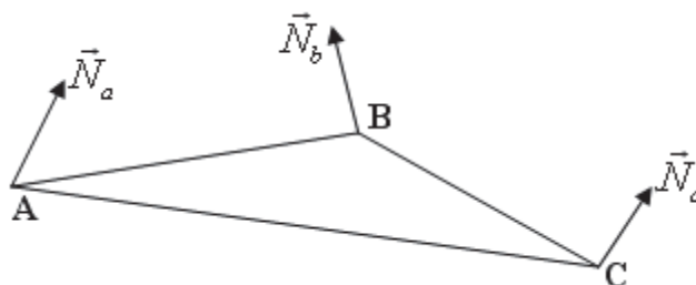
Рисунок 1 – вектори нормалей у вершинах трикутника
