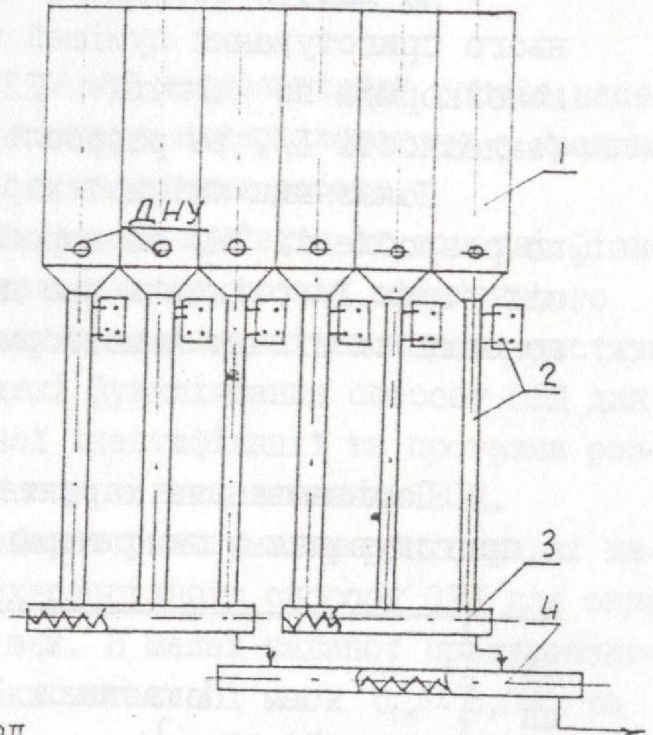
Мал.10. Принципова схема ТНС
