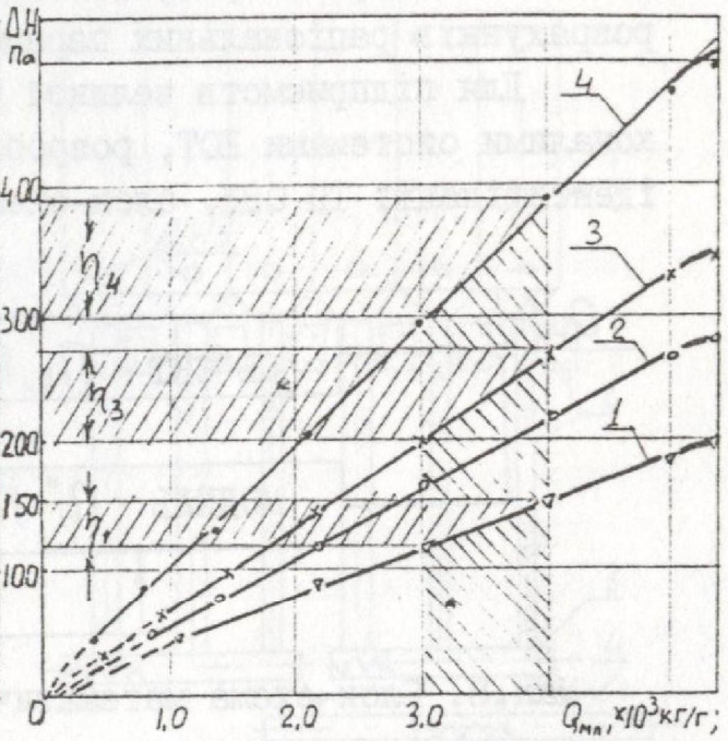
Мал.5. Аналіз метрологічної характеристики ОВД при різних величинах діаметра його камери
