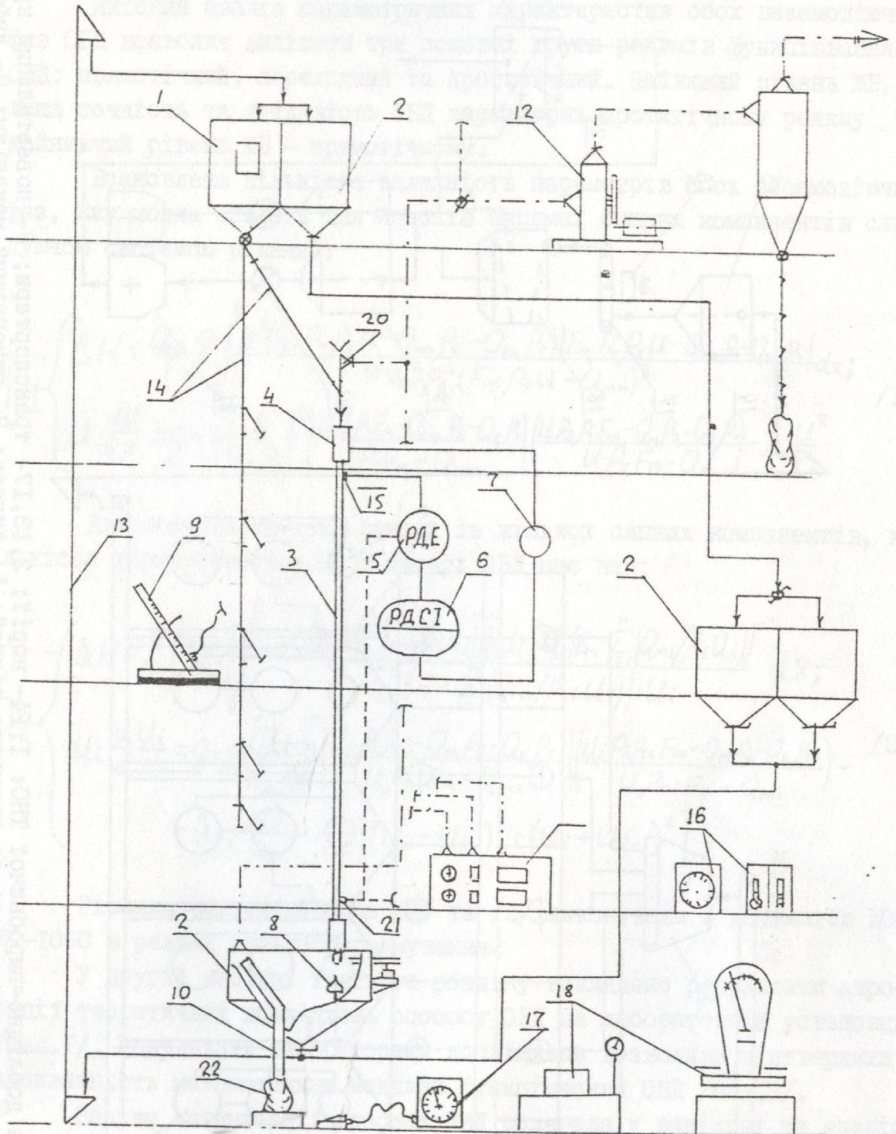
Мал. I. Схема лабораторної установки дослідження ОВД
