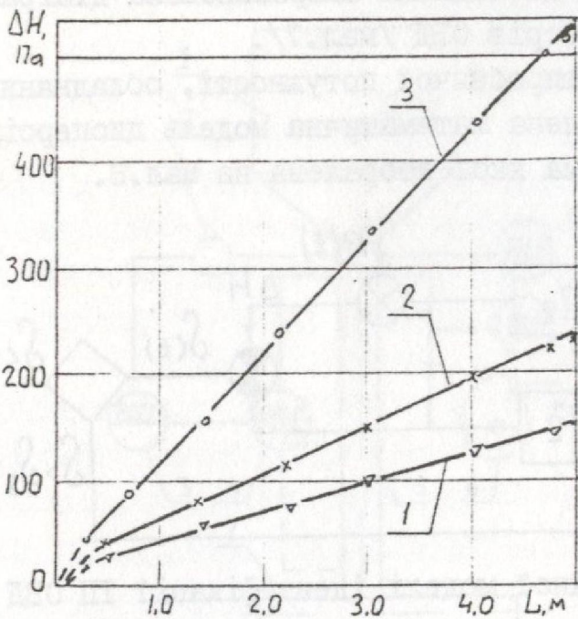
Мал.4. Аеродинамічна характеристика камери ОВД різних довжин:
