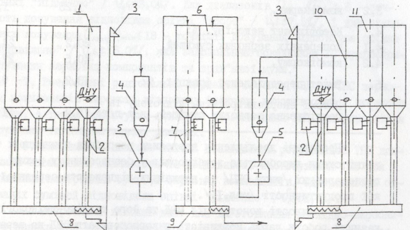
Мал.11. Принципова схема технології виробництва комбікормів без- перервним способом з застосуванням розробленої ТНС
