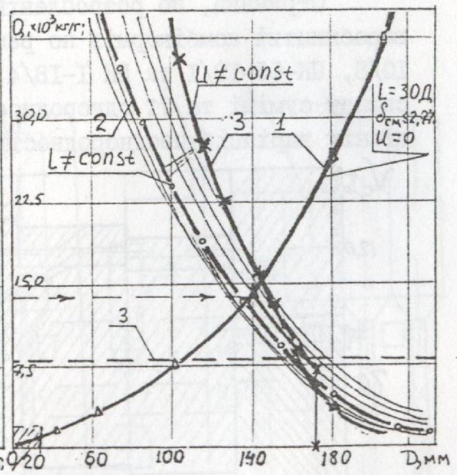
Мал. 7. Діаграма розрахунку раціональних параметрів ОВД
