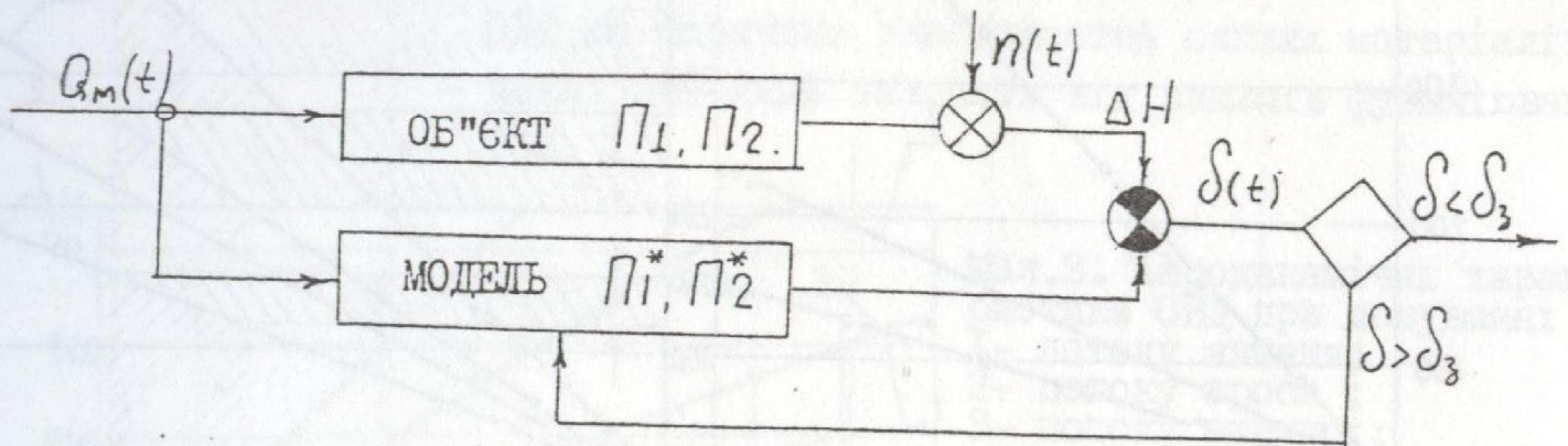
Мал.8. Блок-схема математичної моделі ідентифікації ТП ОВД
