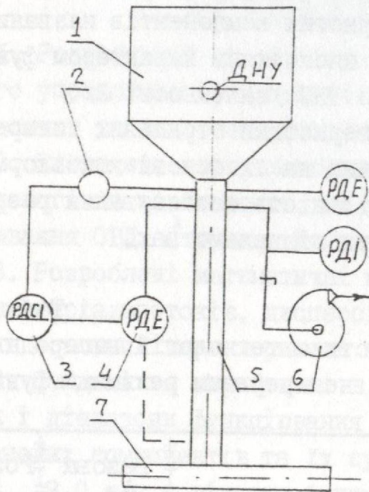
Мал.9. Схема функціонування ОВД
