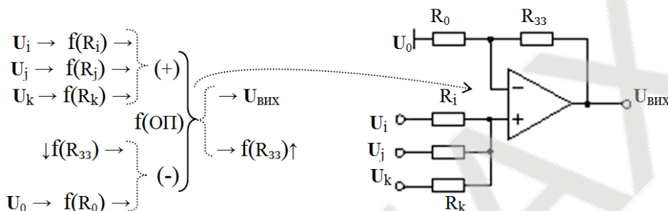
Рис. 4. Графоаналітична модель неінвертуючого суматора
