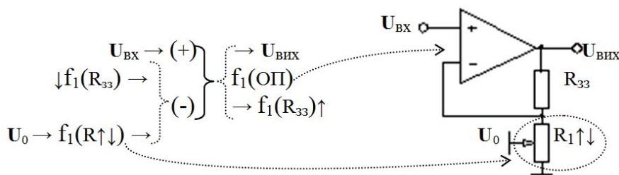
Рис. 3. Графоаналітична модель функціональної структури підсилювача
