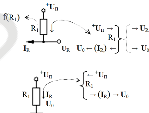
Рис. 5. Графоаналітичні моделі функціональної структури резистора
