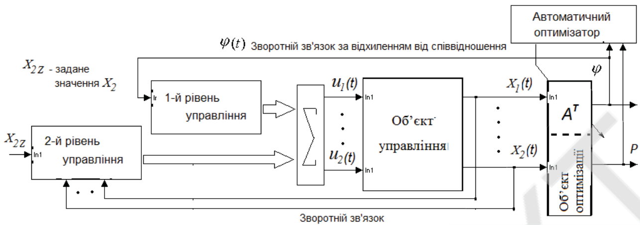
Рисунок 1. Структурна схема багаторівневої координувальної системи автоматичного управління, що забезпечує узгодження перехідних процесів
