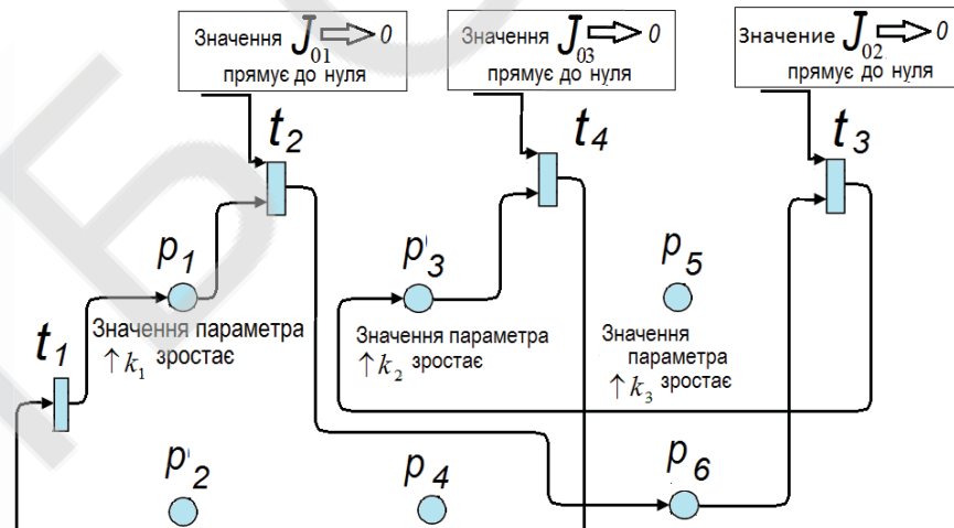
Рисунок 2. Фрагмент мережі Петрі, що представляє процес настроювання багаторівневої системи управління
