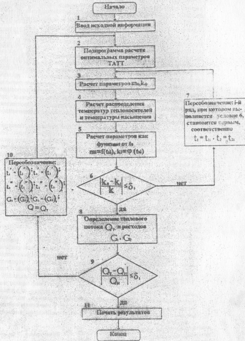
Рис. 3 Блок-схема проектного расчета ТАТТ с элементами оптимизации
