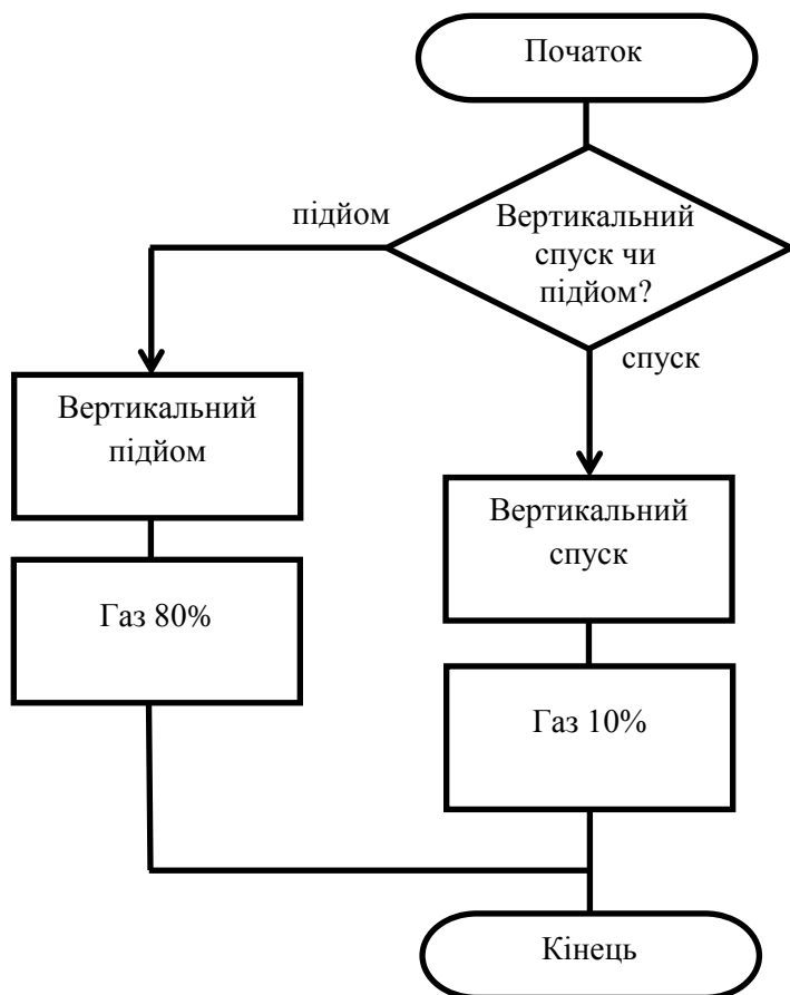
Рис. 1.12 – Алгоритм підйому-спуску квадрокоптера
