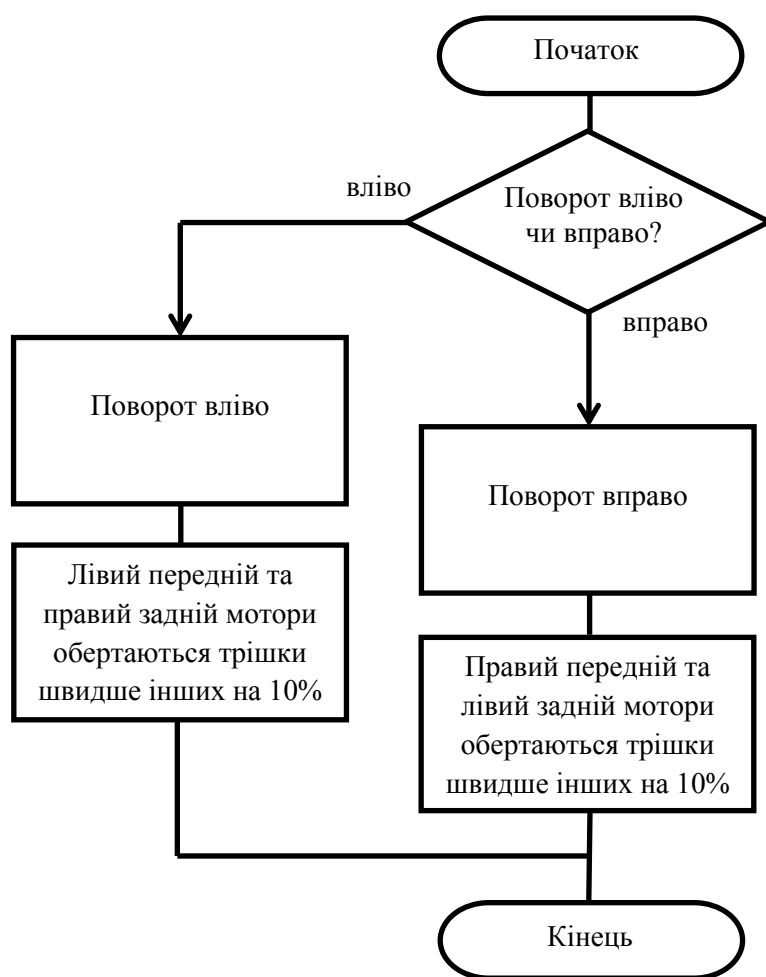
Рис. 1.13 – Алгоритм повороту вліво-вправо квадрокоптера
