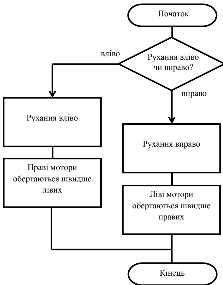
Рис. 1.15 – Алгоритм рухання вліво-вправо квадрокоптера
