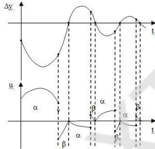
Рис. 3. Часові діаграми ПП СЗС у режимі перемикання
