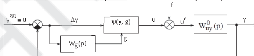
Рис. 1. Структурна схема розглядуваної СЗС
