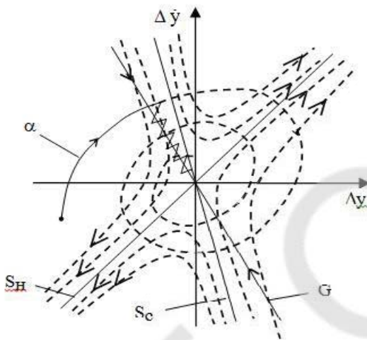
Рис. 2. Фазовий портрет ПП СЗС у режимі перемикання
