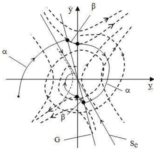
Рис. 2. Фазовий портрет ПП СЗС у режимі перемикання
