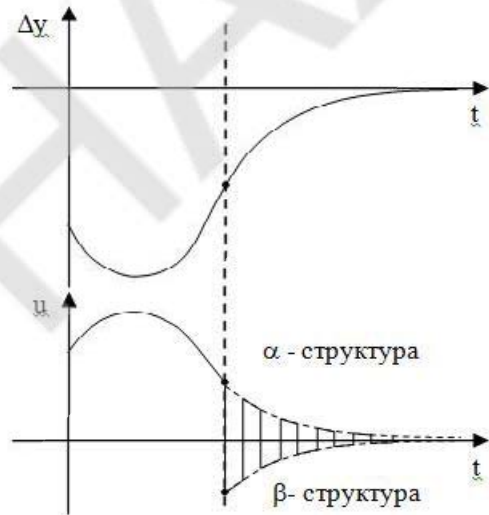
Рис. 5. Часові діаграми ПП СЗС у режимі ковзання
