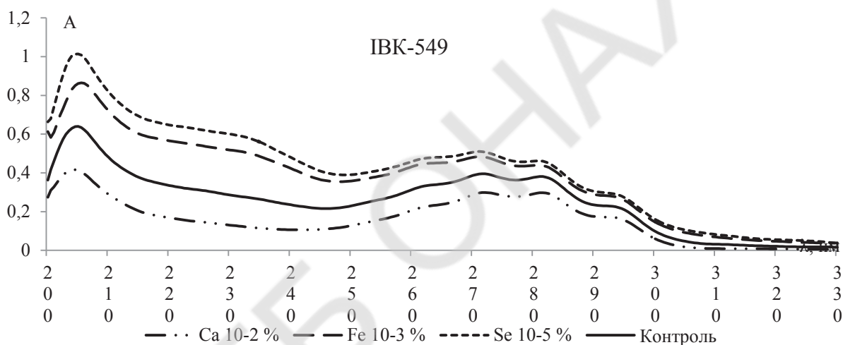
Рис. 2 – УФ-спектри гексанових екстрактів штаму IBK-549 Pl.ostreatus (субстрат – соняшникове лушпиння)
