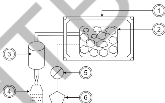
1 - резонаторна камера; 2 - радіо прозора ємність з сировиною; 3 - холодильник-дистилятор; 4 - ємність для збору рідини; 5 - вакууметр; 6 - вакуум-насос.
