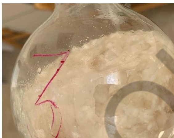
Рис. 2 – Суміш білків після гідролізу і осадження сіллю.
