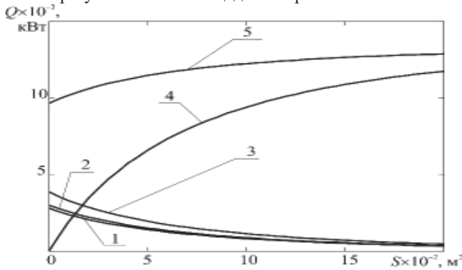
1 – на первом теплообменном аппарате; 2- на втором теплообменнике; 3- на третьем; 4 – на четвертом; 5- общая мощность рекуперации теплоты в новой теплообменной системе.
