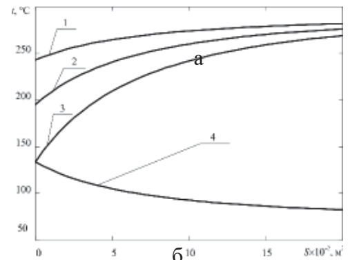
а) - изменение температуры холодного теплоносителя. 1- температура входа в 4й теплообменник, 2- в 3й, 3- во 2й, 4 в 1й; б) - горячего теплоносителя в зависимости от величины площади поверхности теплообмена нового теплообменника. 1- температура выхода из 1го теплообменника, 2- из 2го, 3- из 3го, 4 из 4го.
