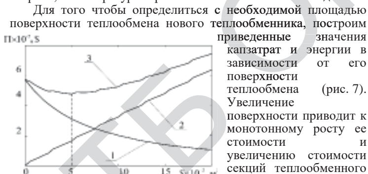
1 – годовая стоимость энергии; 2- приведенные капитальные затраты; 3- общая приведенная стоимость проекта реконструкции.
