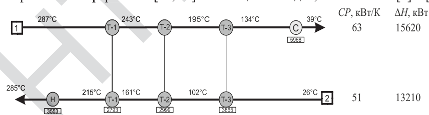
Рис. 1. Сеточная диаграмма двухпоточковой задачи
