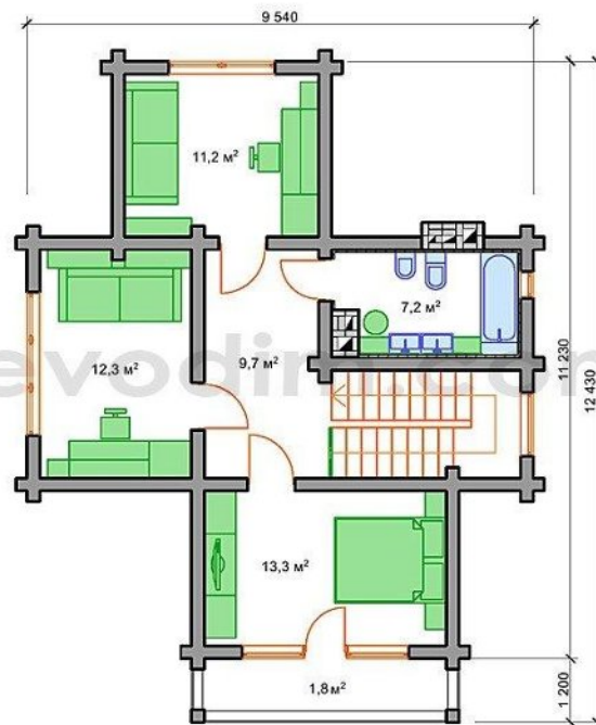
Рис. 2.5 - Проект котеджу класу "апартамент"
