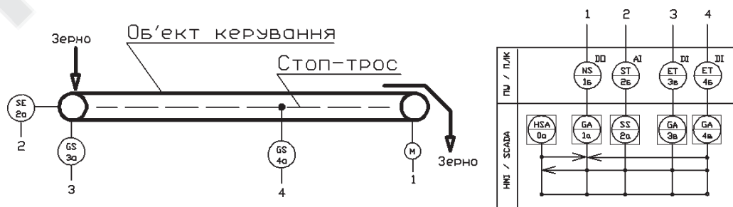
Рис. 1. Фрагмент схеми керування стрічковим конвеєром.
