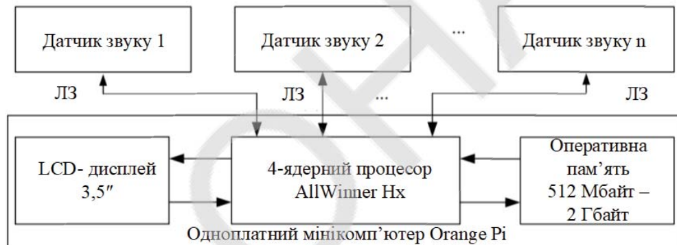
Рисунок 4 – Структурна схема багатодатчикової системи пасивної акустичної локації
