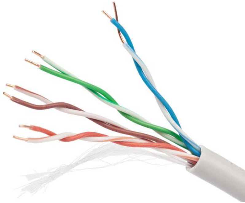
Рисунок 1.9 Мідний кабель
