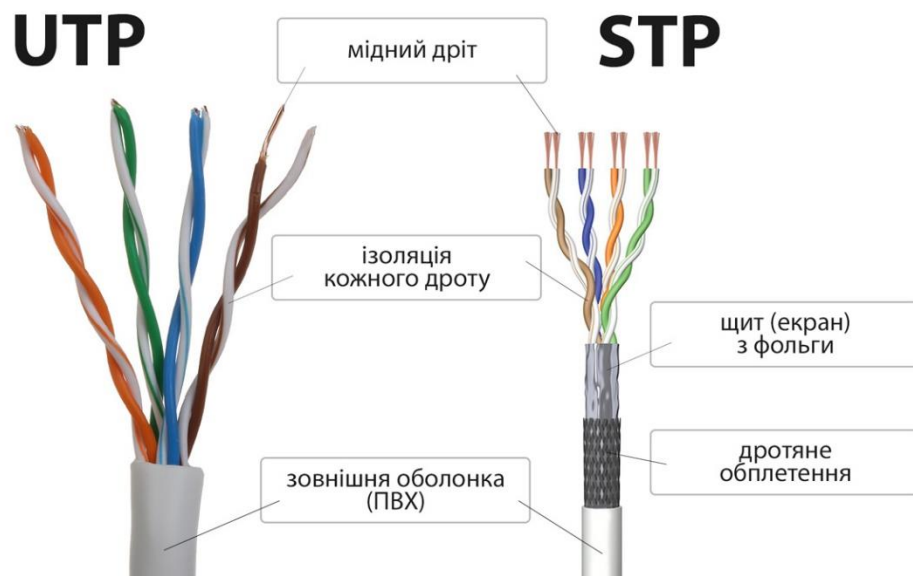
Рисунок 1.15 Відмінності між кабелями UTP та STP витої пари
