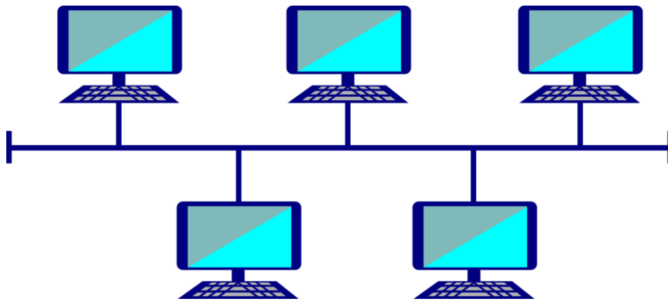
Рисунок 1.4 Топологія «Шина»
