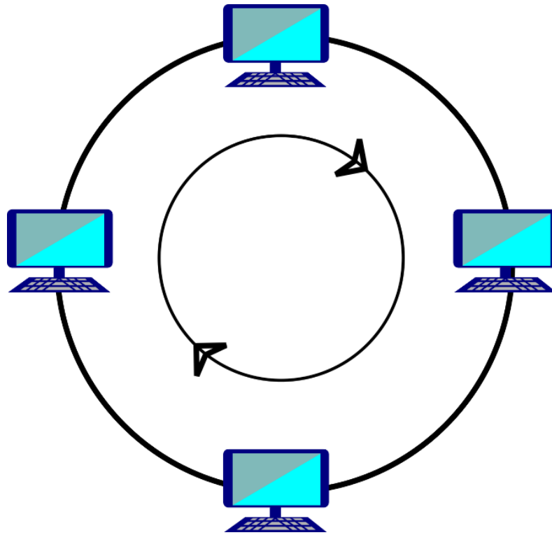
Рисунок 1.6 Топологія «Кільце»
