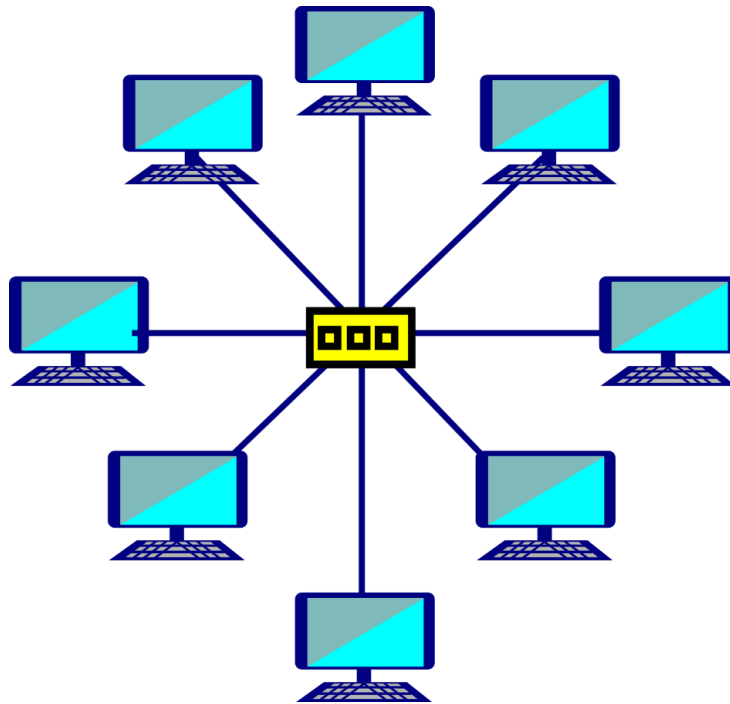
Рисунок 1.5 Топологія «Зірка»
