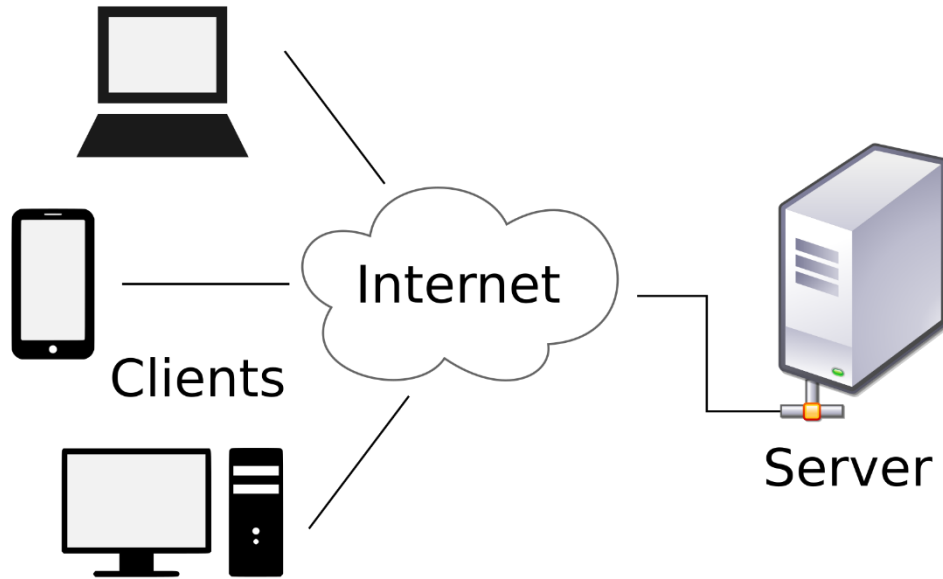
Рисунок 1.3 Модель клієнт/сервер
