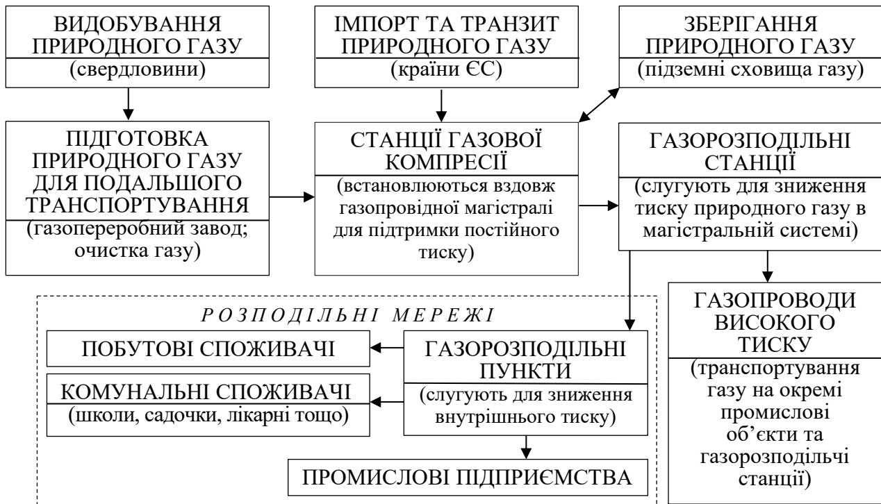
Рис. 1. Схема видобування, імпорту, підготовки, збереження, розподілу, а також транспортування природного газу в Україні
