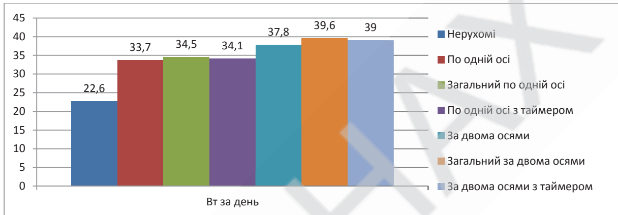
Рисунок 4. Результати проведених експериментів за червень
