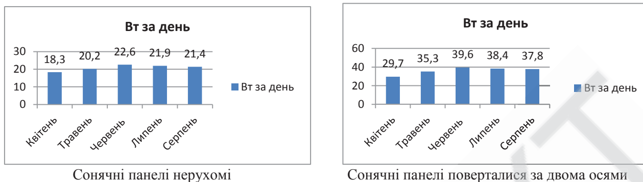
Рисунок 1. Значення вихідної потужності
