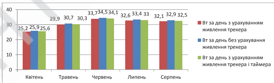
Рисунок 2. Порівняння трьох різних видів експерименту при обертанні панелей по одній осі
