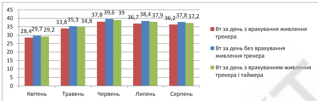
Рисунок 3. Порівняння трьох різних видів експерименту при обертанні панелей за двома осями
