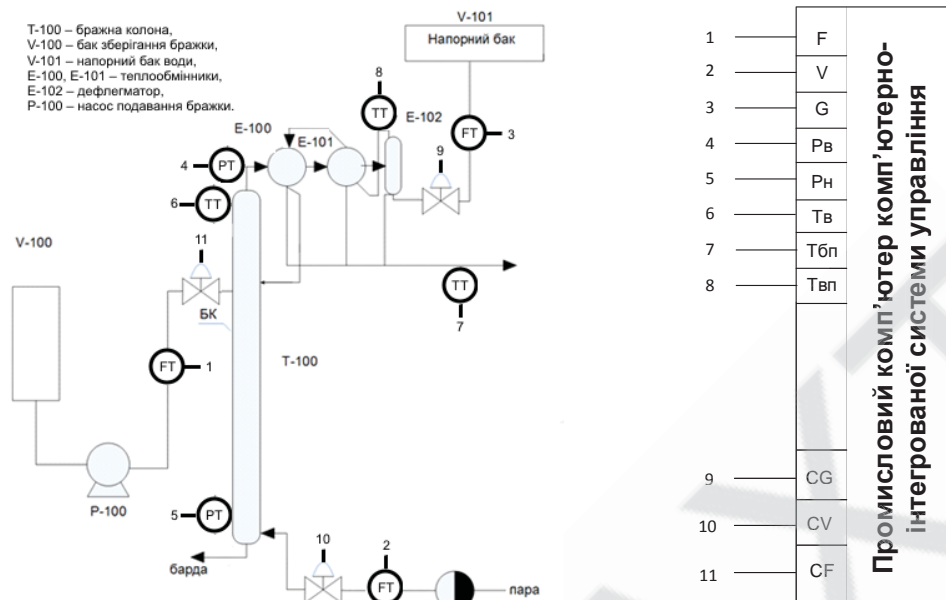
Рисунок 1 – Технологічна схема бражної колони
