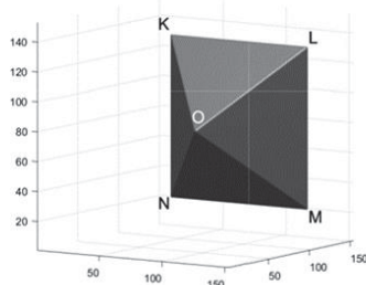
Рисунок 5 - Два типа трехмерных углов, вершина O является центром массива. (а) Фигура OKLMN – пирамида, (б) фигура OABCDEF – октант.
