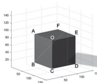
Рисунок 5 - Два типа трехмерных углов, вершина O является центром массива. (а) Фигура OKLMN – пирамида, (б) фигура OABCDEF – октант.
