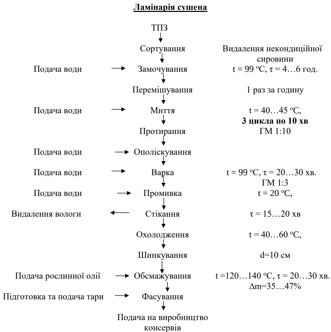
Рис. 3.5 - Технологічна схема підготовки ламінарії сушеної для виробництва салатів
