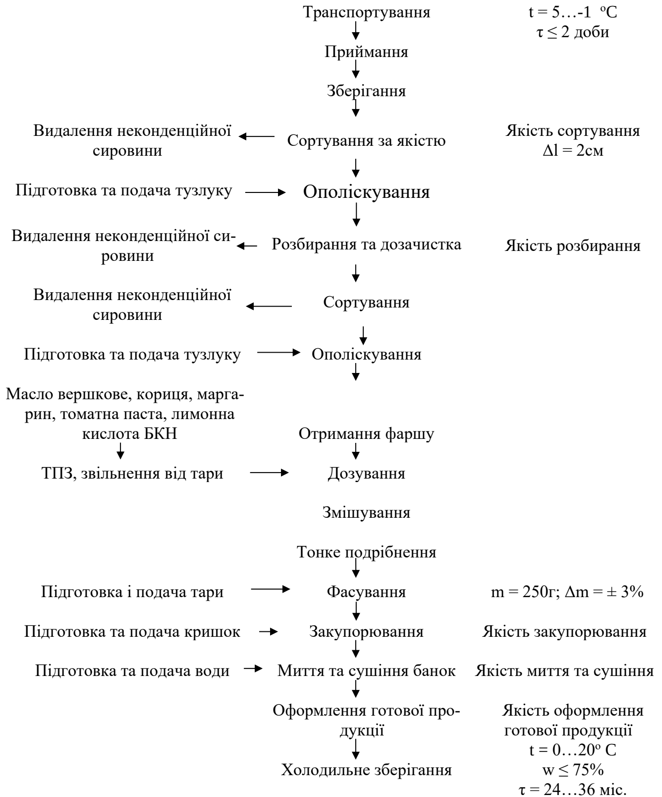
Рис. 3.2 - Технологічна схема виробництва пасти «Русалонька» з оселедцю антілаптичного.
