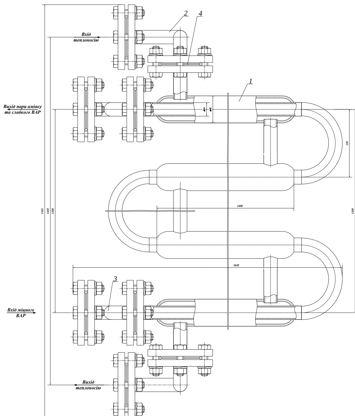
Рис. – Генератор АТТ типу «труба в трубі»:
