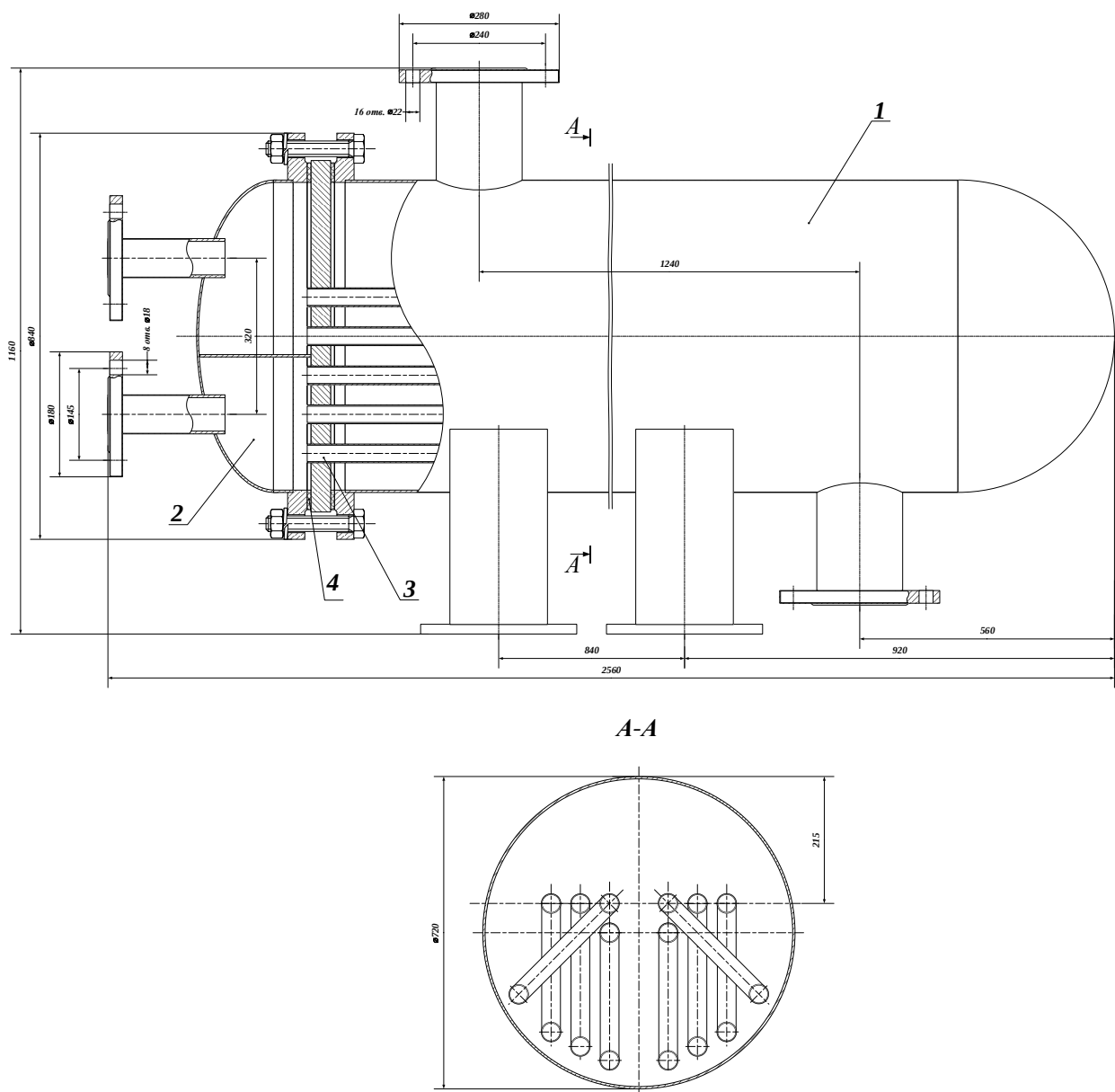
Рис. – Кожутрубный генератор АТТ: 1 – корпус; 2 – крышка; 3 – трубный пучок; 4 – прокладка
