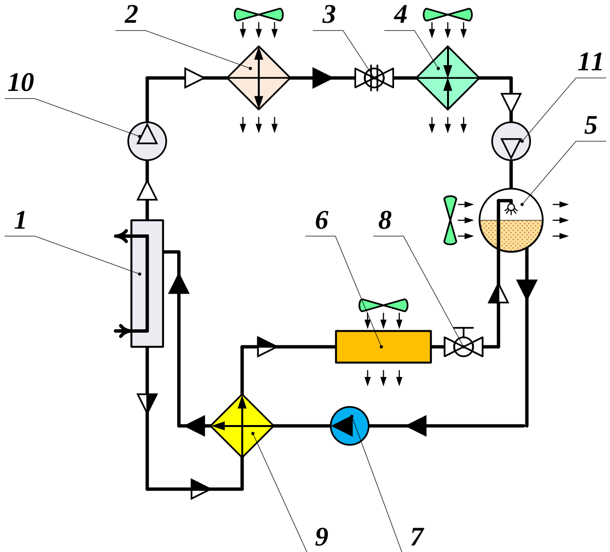
Рис. В.4 – Схема АВТ з двома підтискаючими бустер-компресорами:
