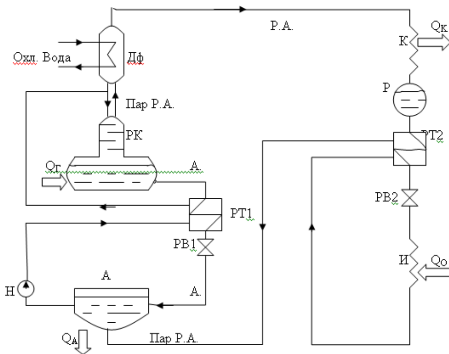
Рис. 1.4 - Схема реальної одноступінчастої абсорбційної холодильної установки:
