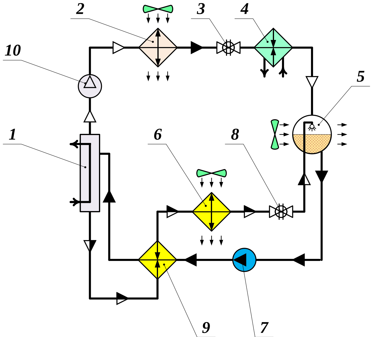
Рис. В.3 – Схема АВТ з підискаючим бустер-компресором:
