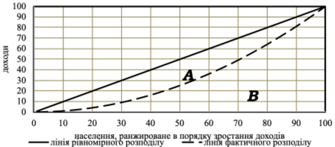
Рис. 3.2. Крива Лоренца (штрихова лінія)
